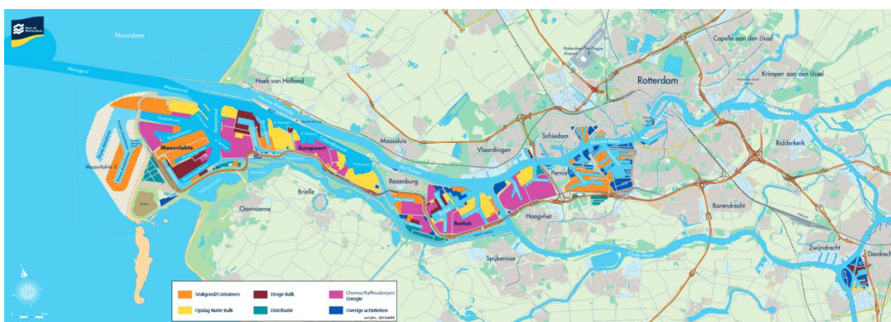
Figuur 2.1 Havengebied Rotterdam opgesplitst naar activiteiten
